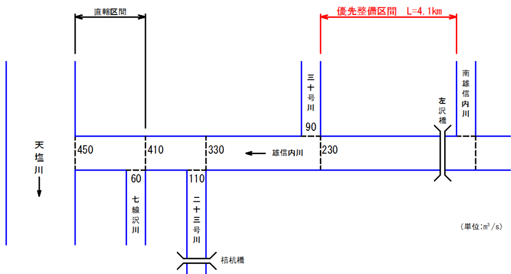
図-3 河川整備計画目標流量配分図
