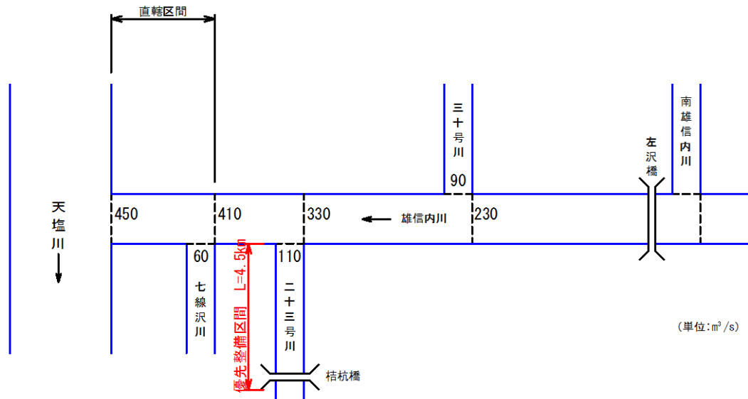
図-4 河川整備計画目標流量配分図
