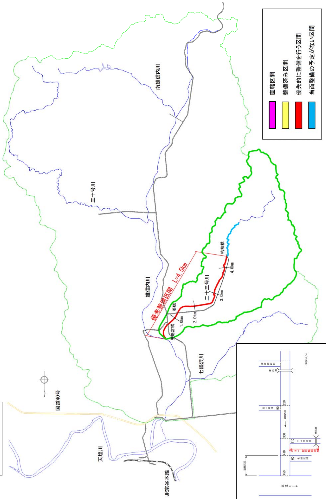
二十三号川 平面図
