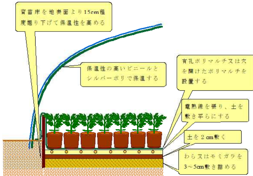
図 育苗床の模式図
