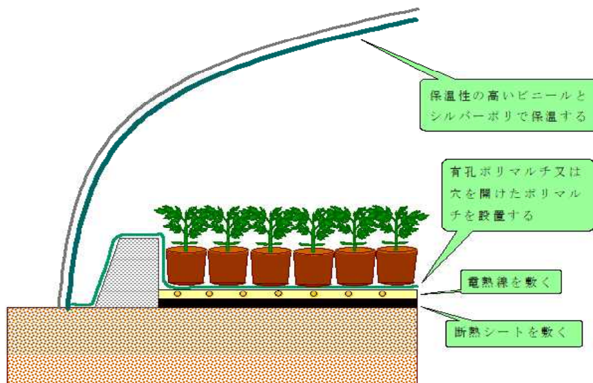
図 育苗床の模式図
