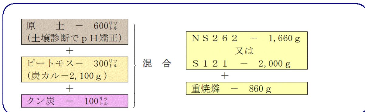
図 促成床土の作り方 (床土を1,000 kg 作り1,250 ポット 分用意する場合)
